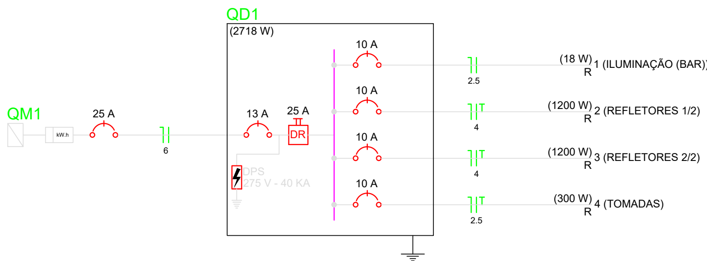
Quadro de Cargas (QD1)
