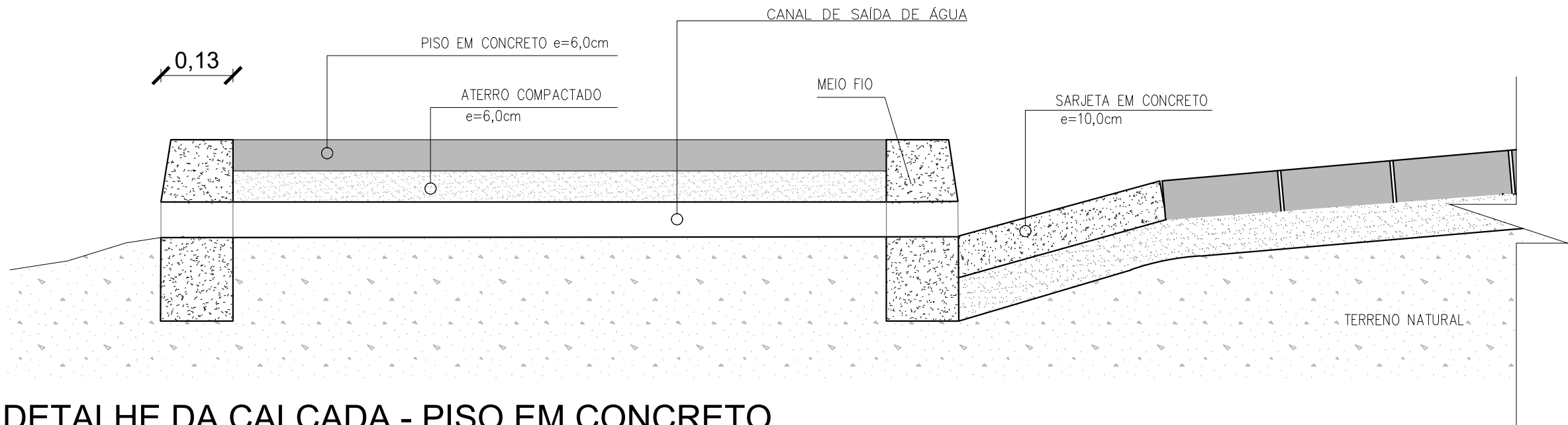
DETALHE DA CALÇADA - PISO EM CONCRETO ESC.1/200
