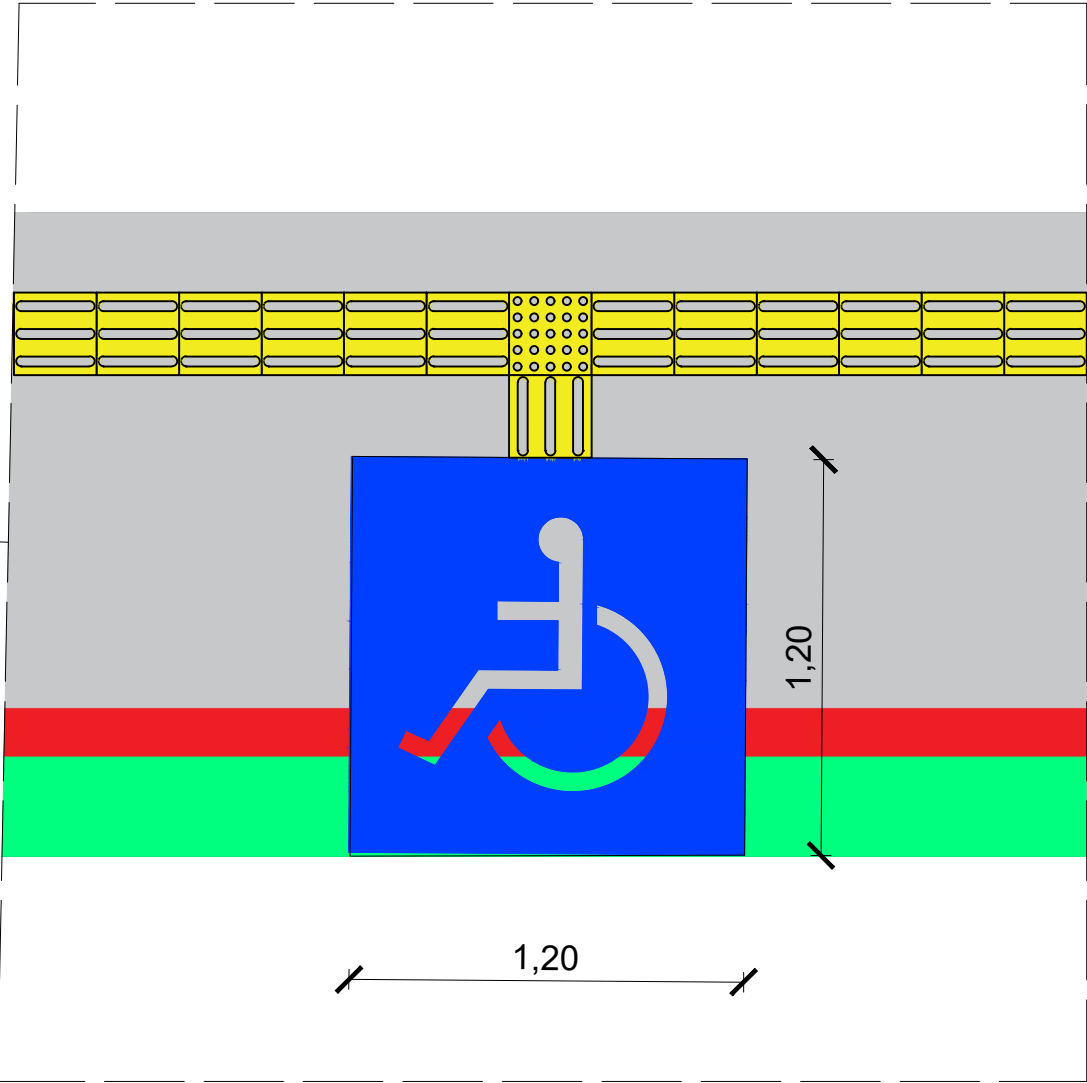
DETALHE RAMPA SEM ESCALA
