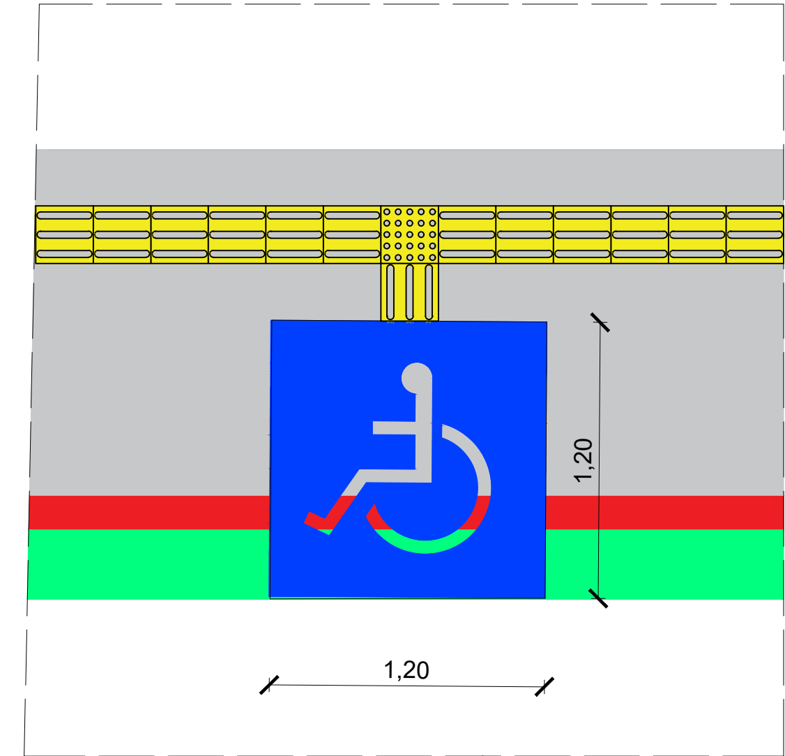
DETALHE RAMPA SEM ESCALA
