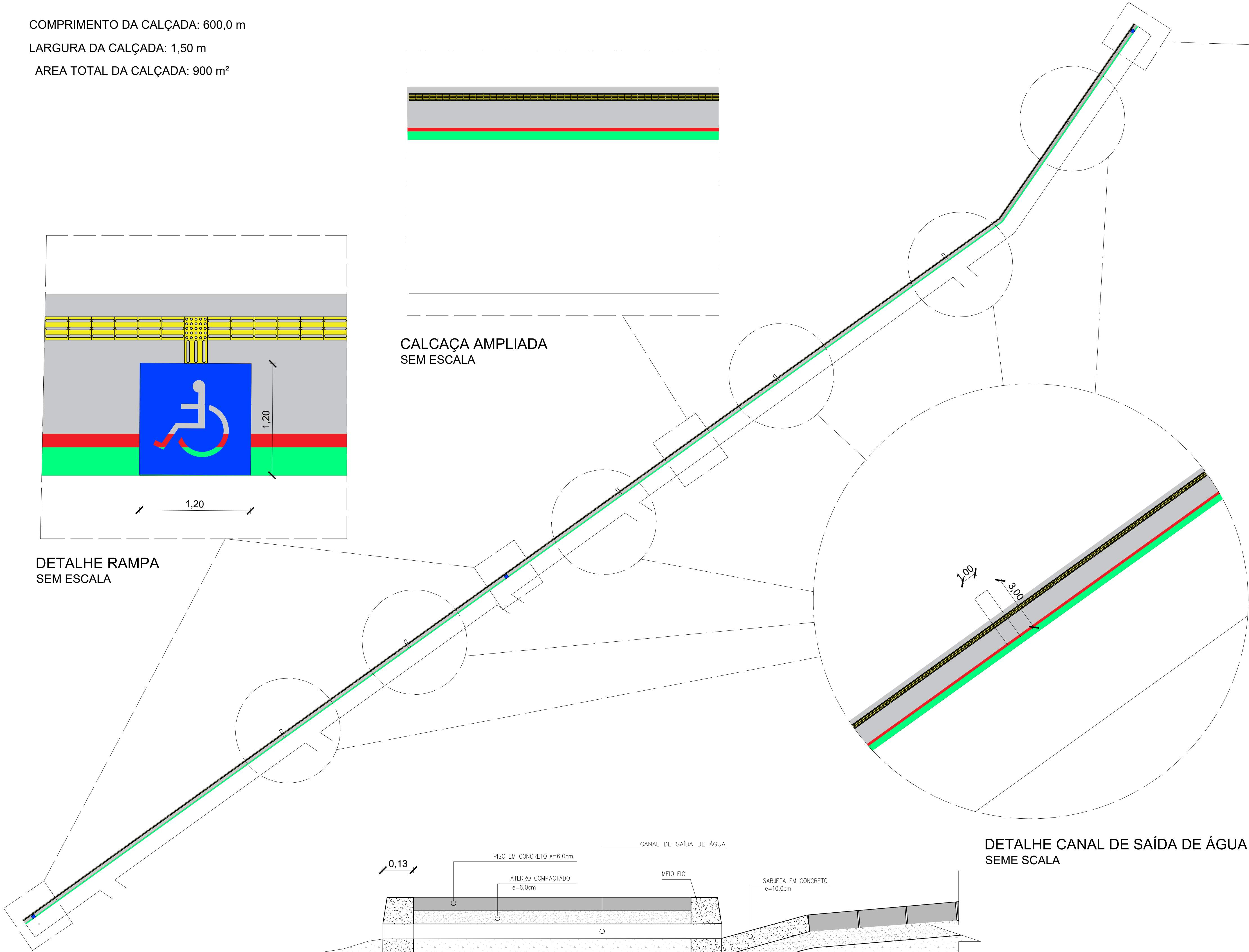
PLANTA BAIXA ESC. 1/750
