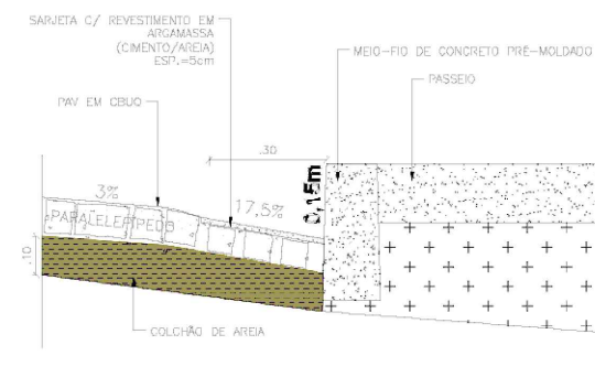
DETALHE SARJETA 1/20
