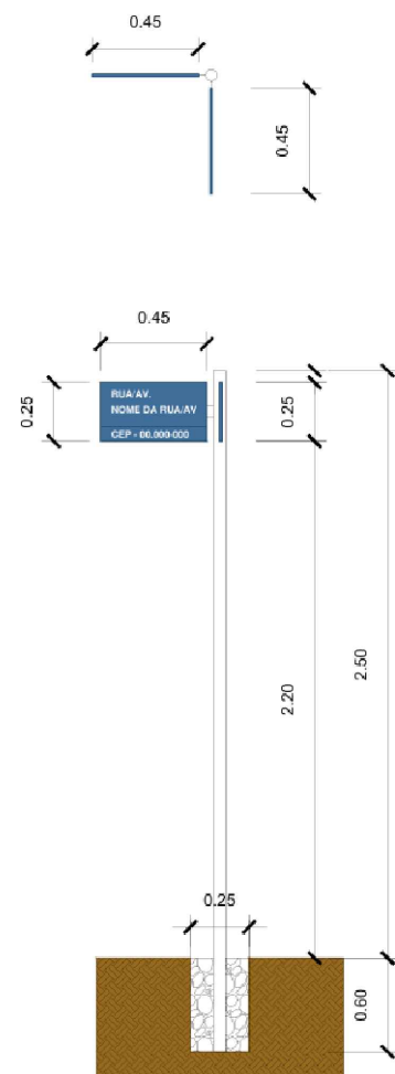
DETALHE PLACA 1/50
