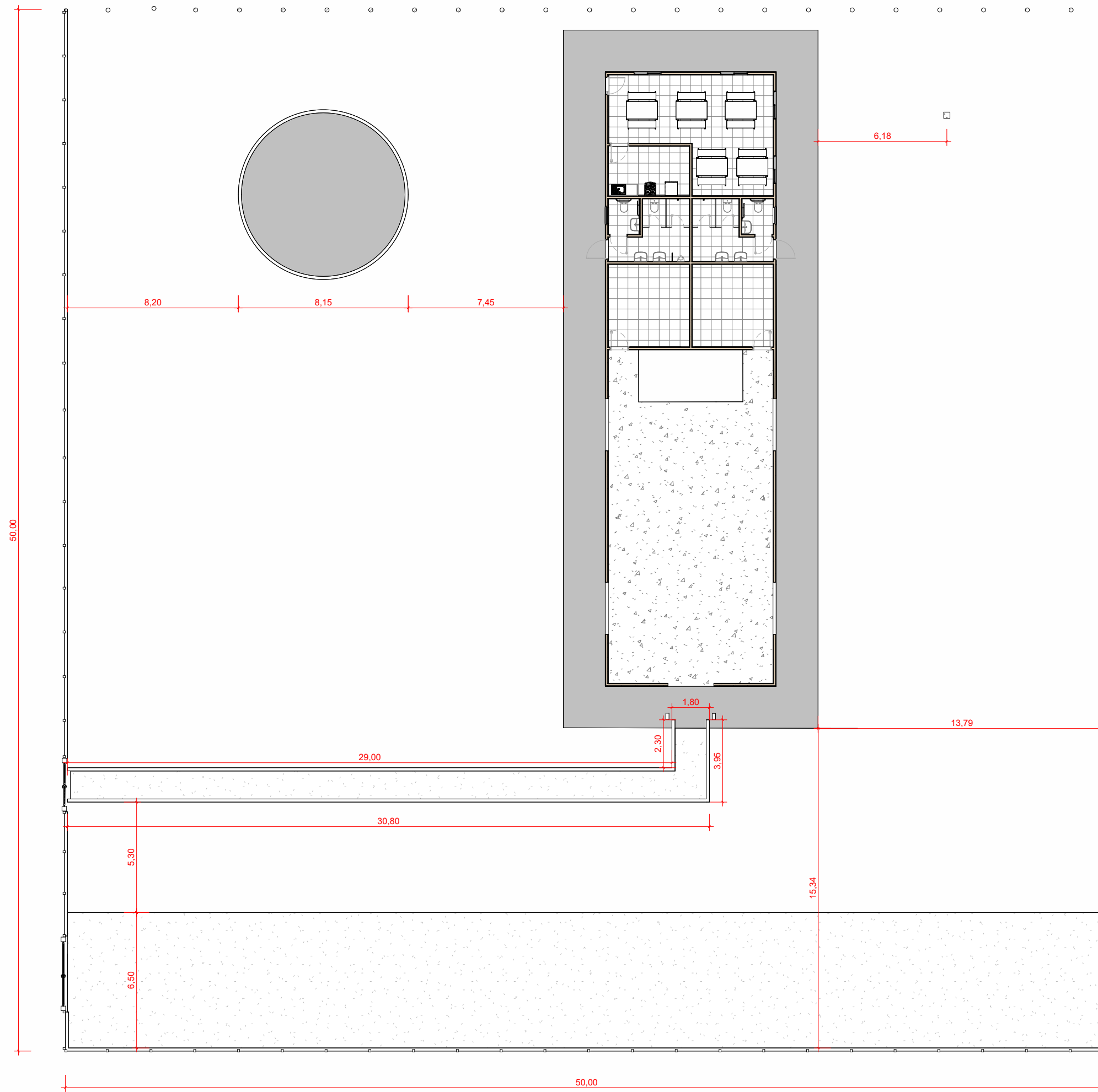
2 Planta Baixa - Geral 1:200
