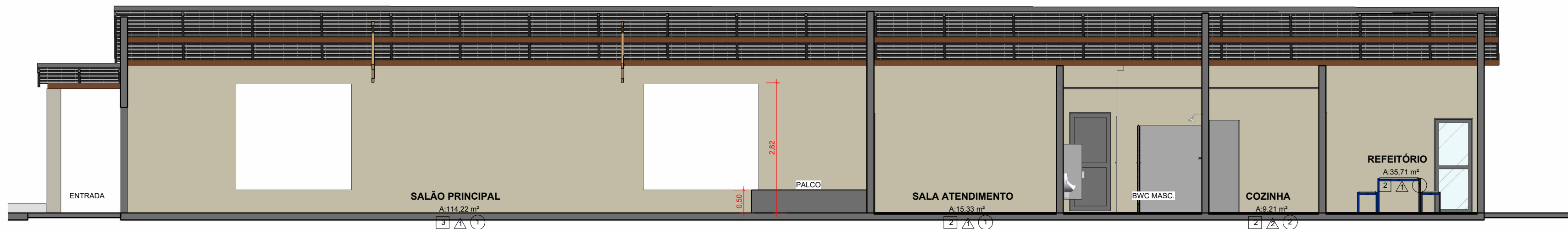
1 Corte A-A 1 : 75
