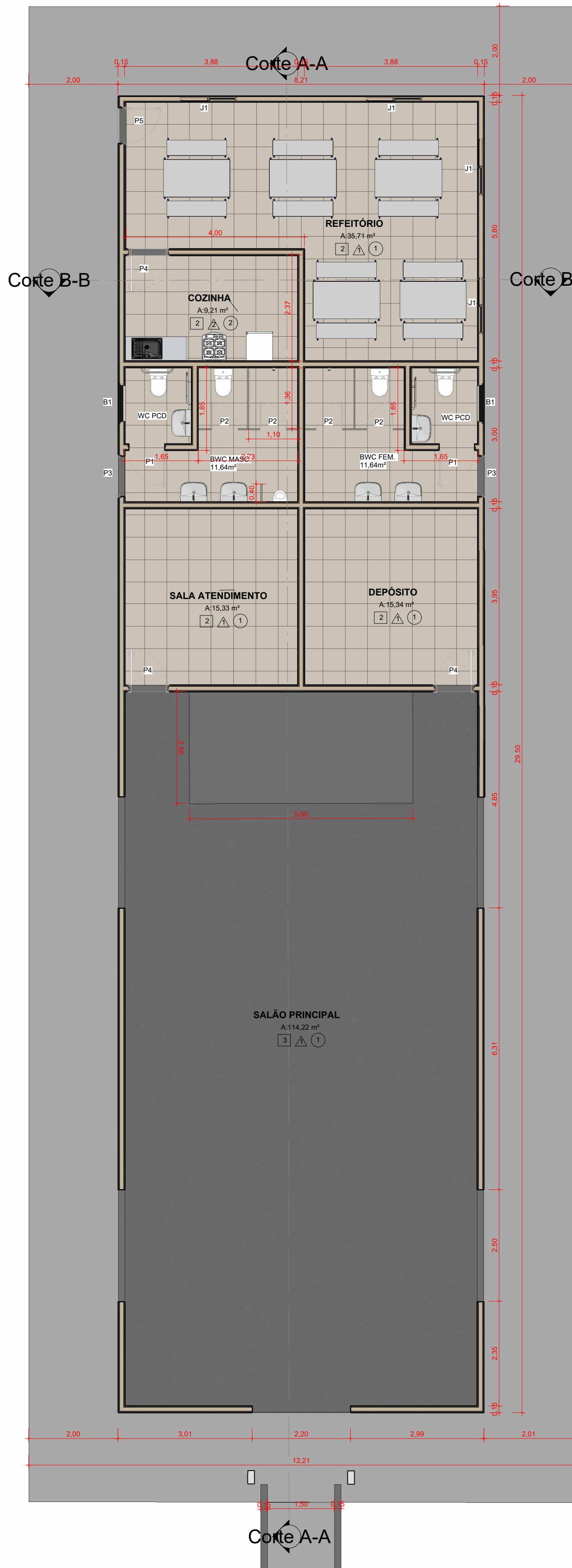
1 Planta Baixa - Salão Principal 1:75
