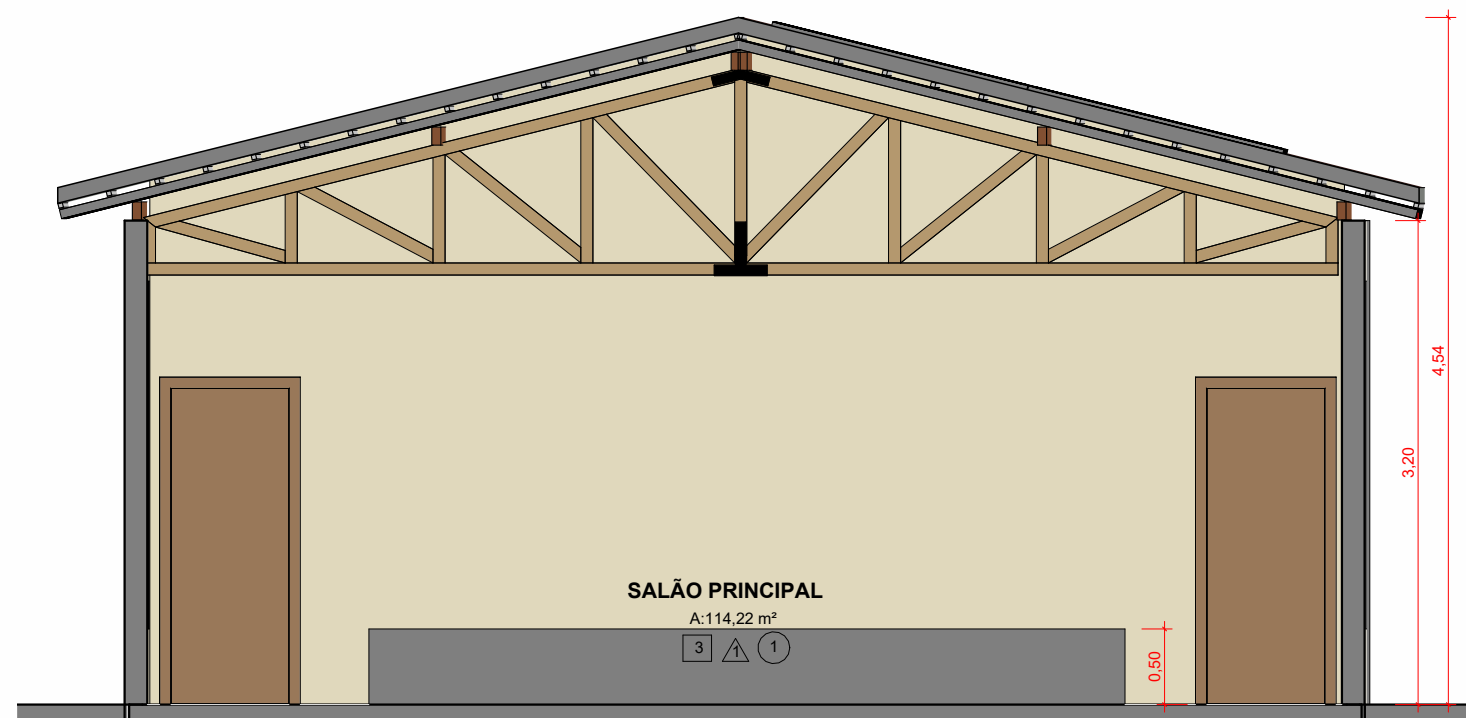
3 Corte C-C 1 : 50
