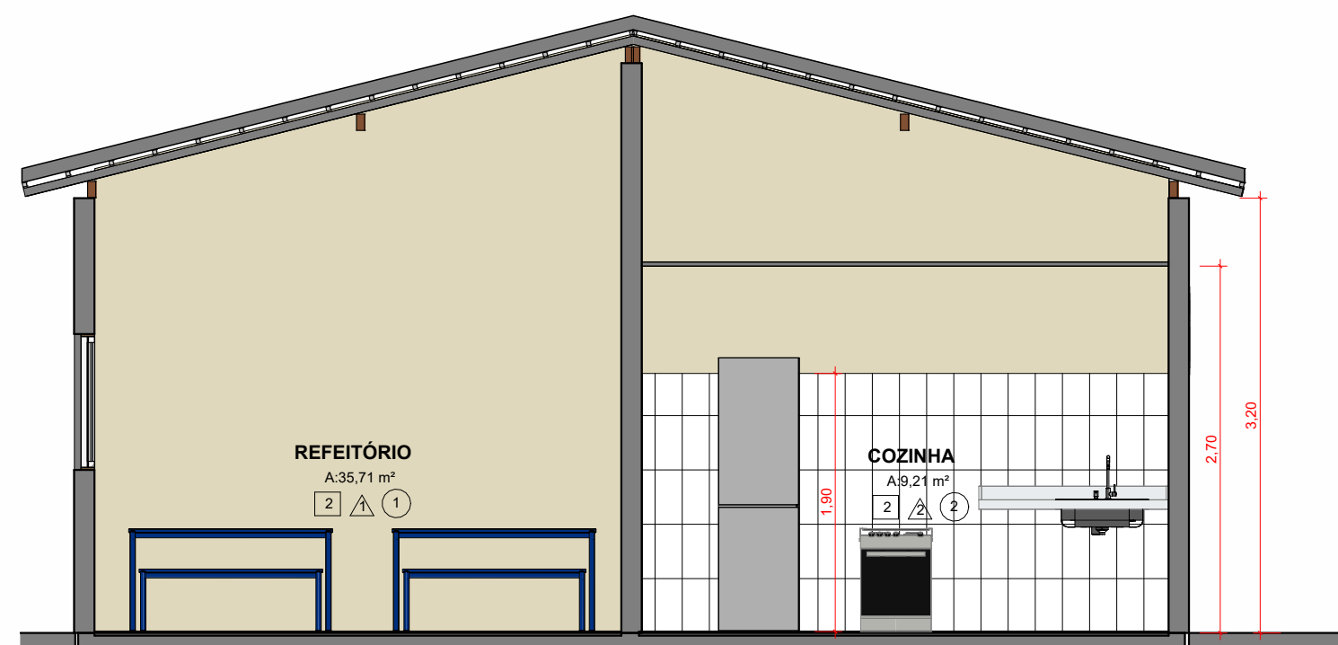
2 Corte B-B 1 : 50
