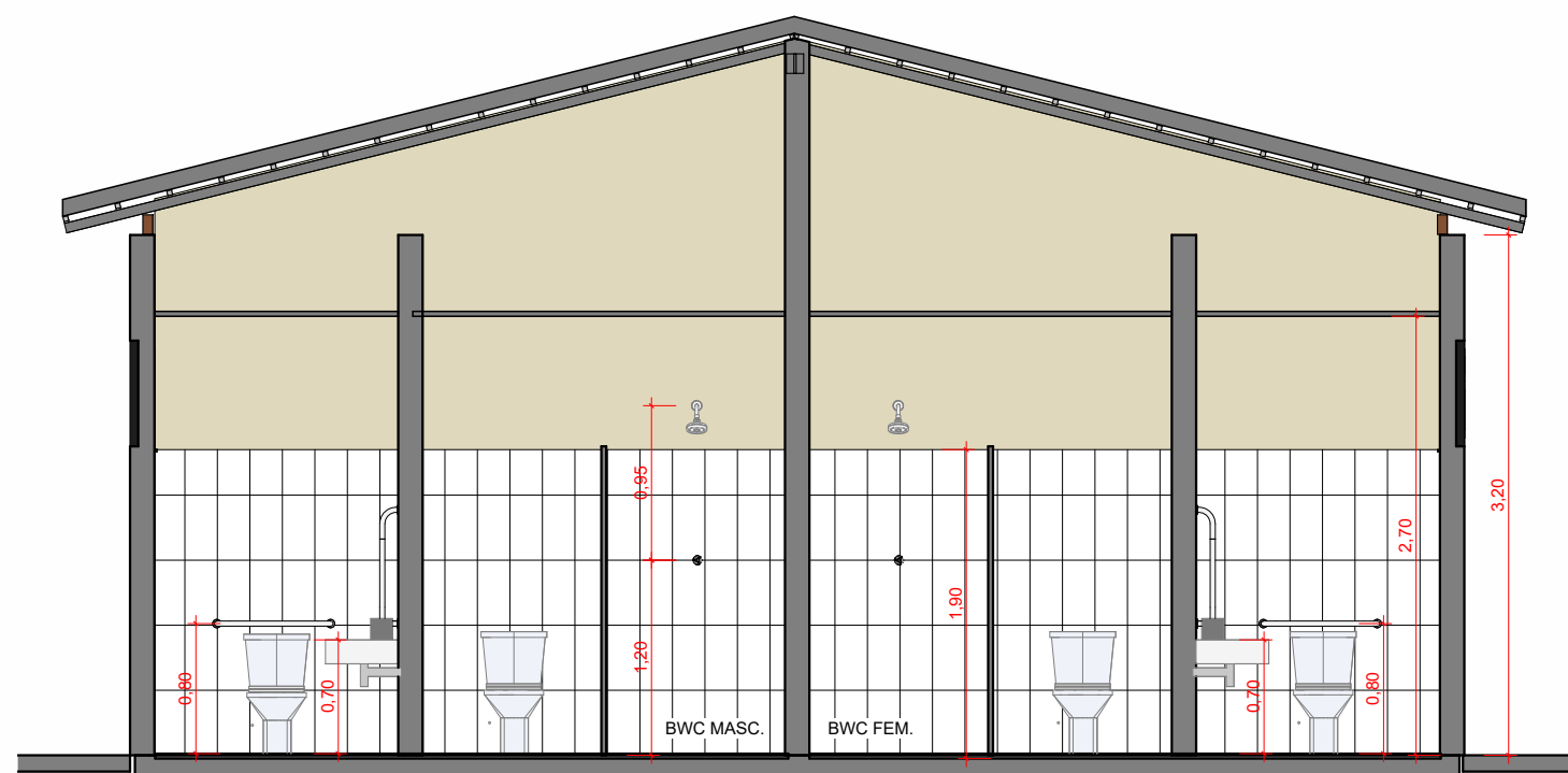
4 Corte D-D 1 : 50
