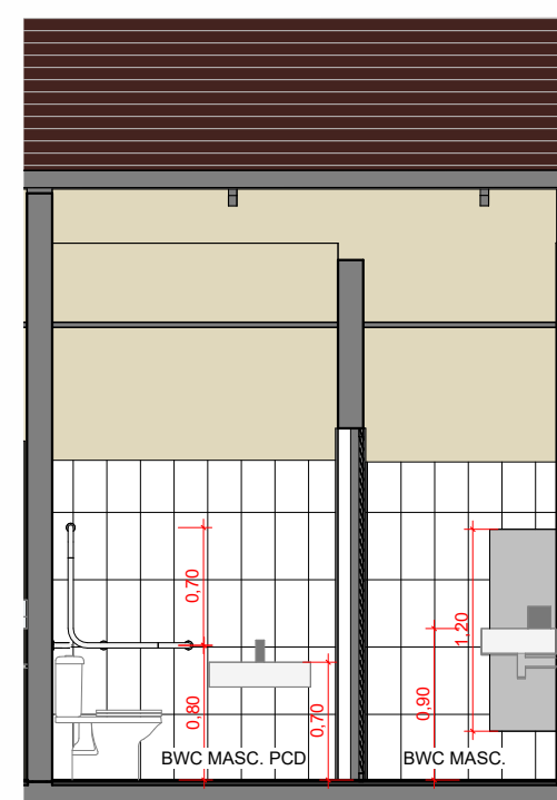
5 Corte E-E 1 : 50
