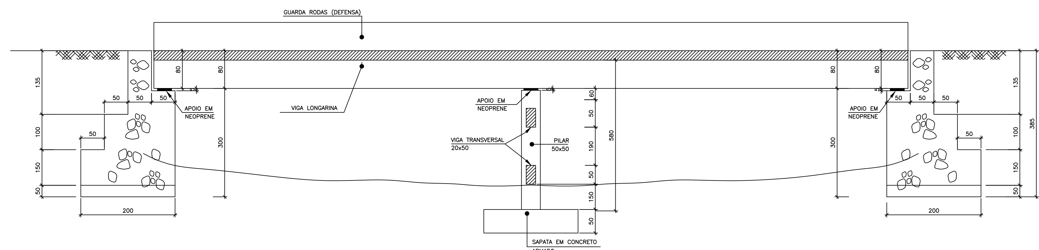
03 CORTE C1 - C1 (LONGITUDINAL)
