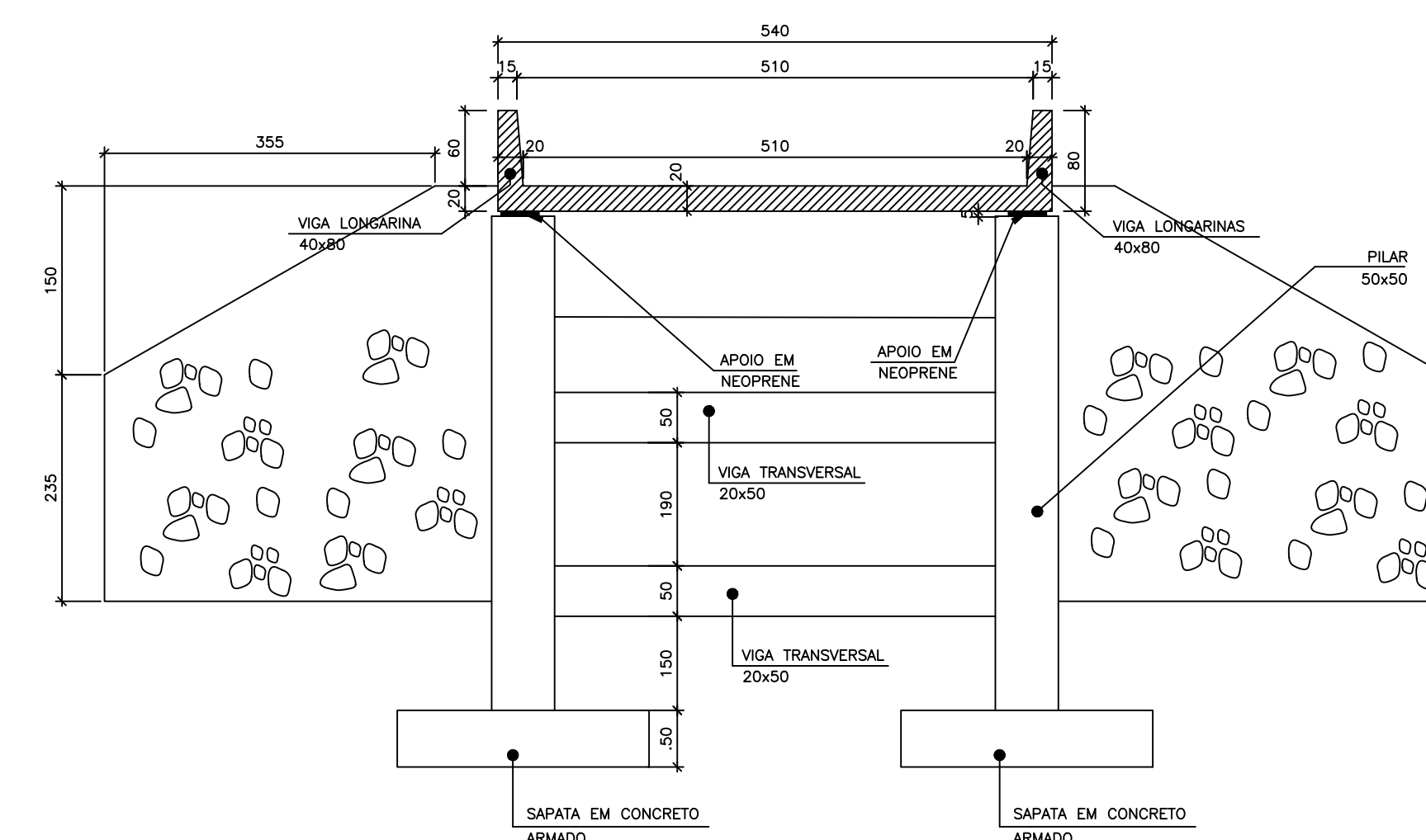
03 CORTE C1 - C1 (LONGITUDINAL)
