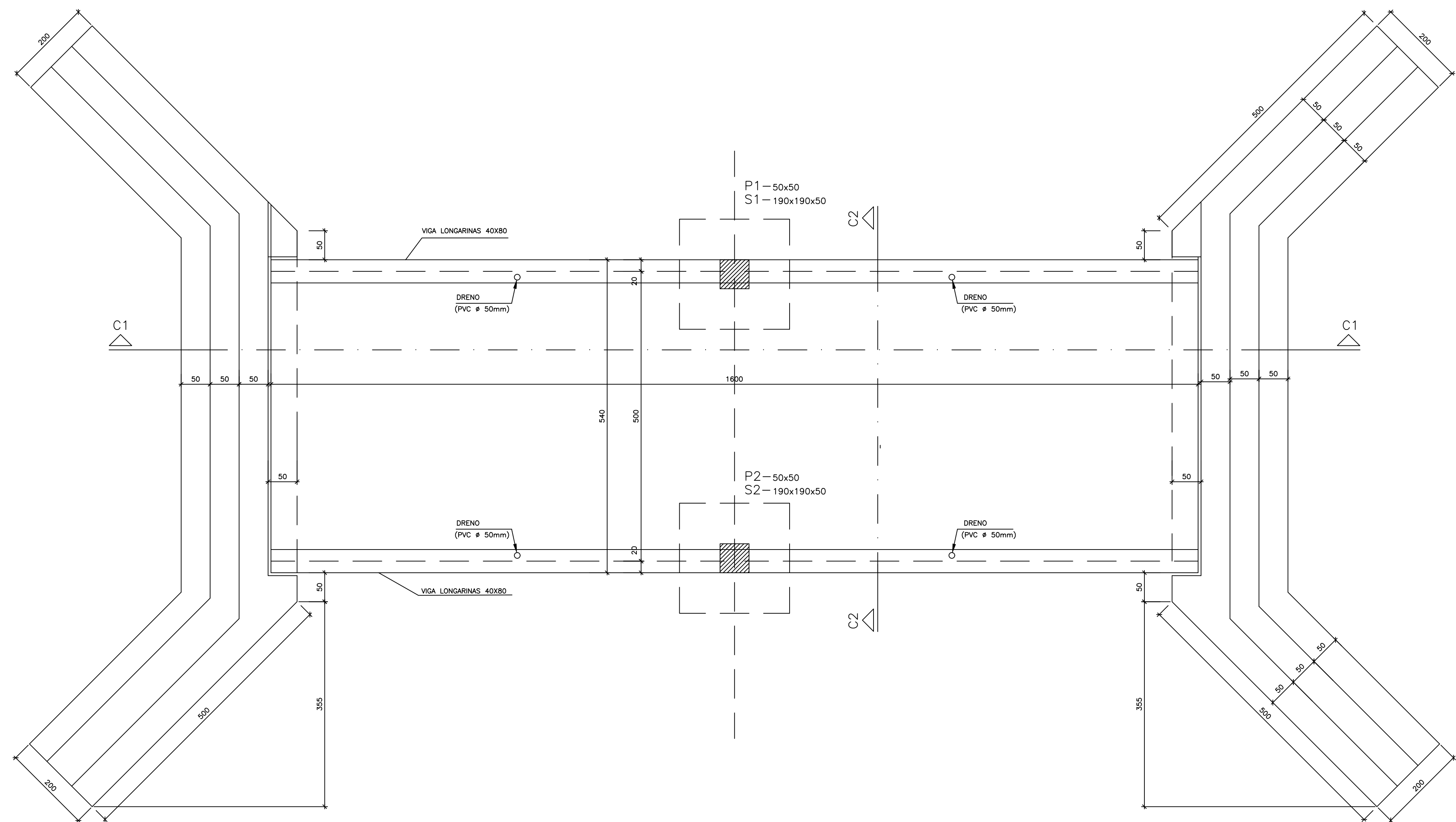
01 VISTA SUPERIOR DA PONTE
