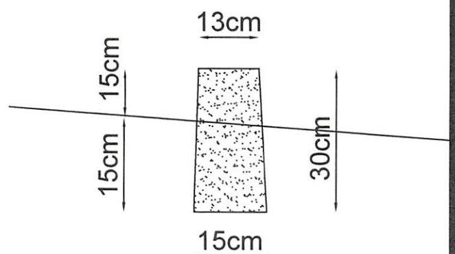
MEIO-FIO DE CONCRETO PRÉ-MOLDADO
