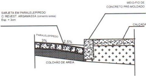
DETALHE - 01
