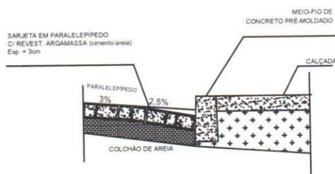
DETALHE - 01
