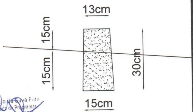
MEIO-FIO DE CONCRETO PRÉ-MOLDADO
