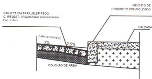
DETALHE - 01
