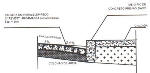
DETALHE - 01
