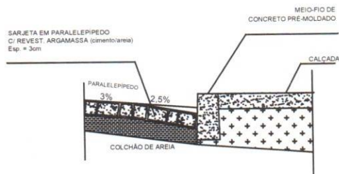
DETALHE - 01
