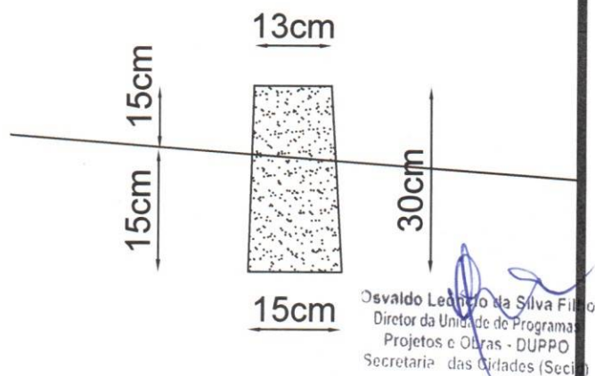
MEIO-FIO DE CONCRETO PRÉ-MOLDADO
