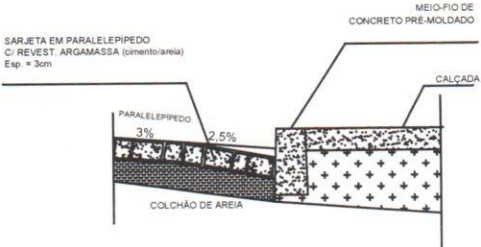
DETALHE - 01
