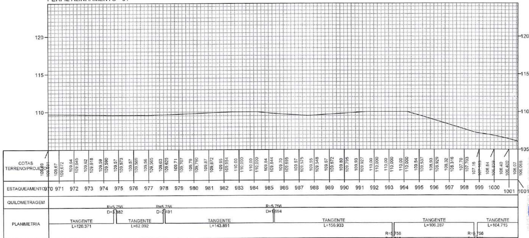
PERFIL ALINHAMENTO - 01
