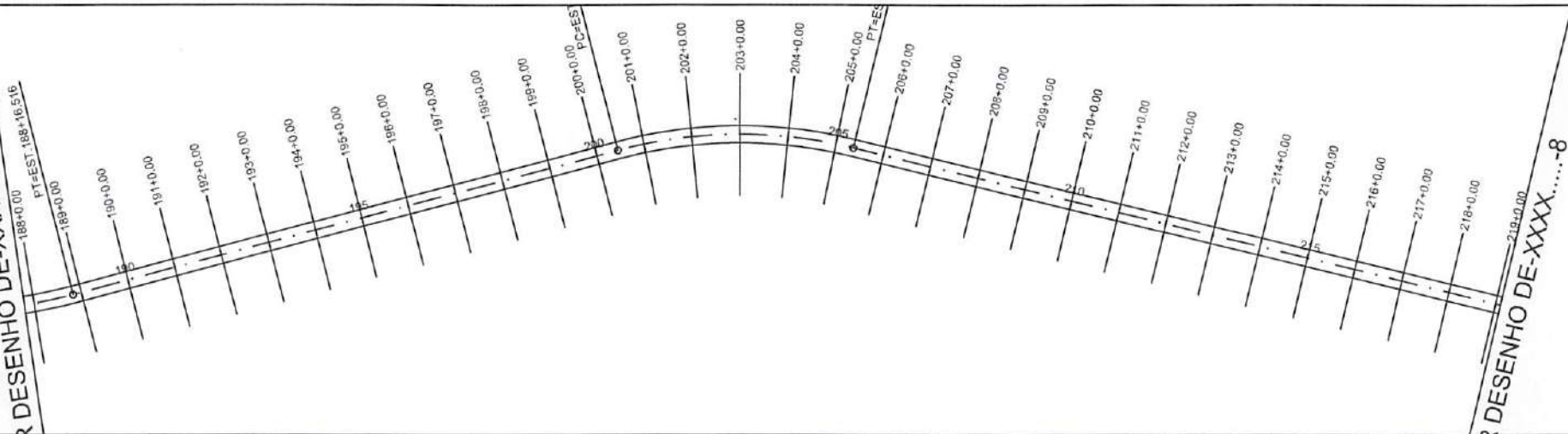
PERFIL ALINHAMENTO - 01
