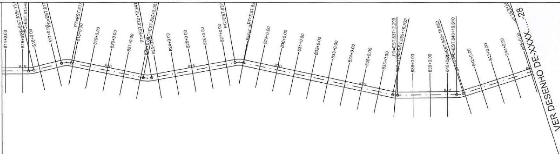
PERFIL ALINHAMENTO - 01
