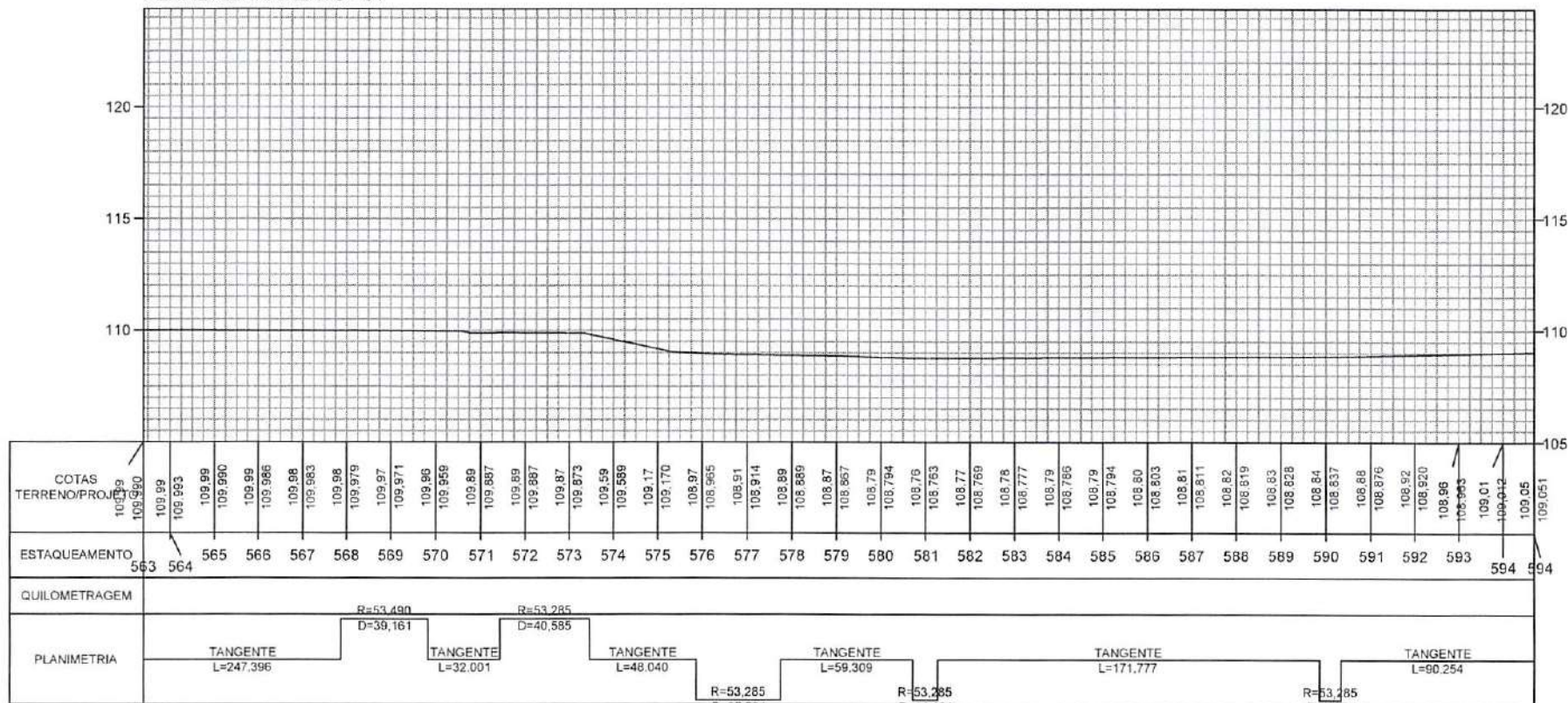
PERFIL ALINHAMENTO - 01
