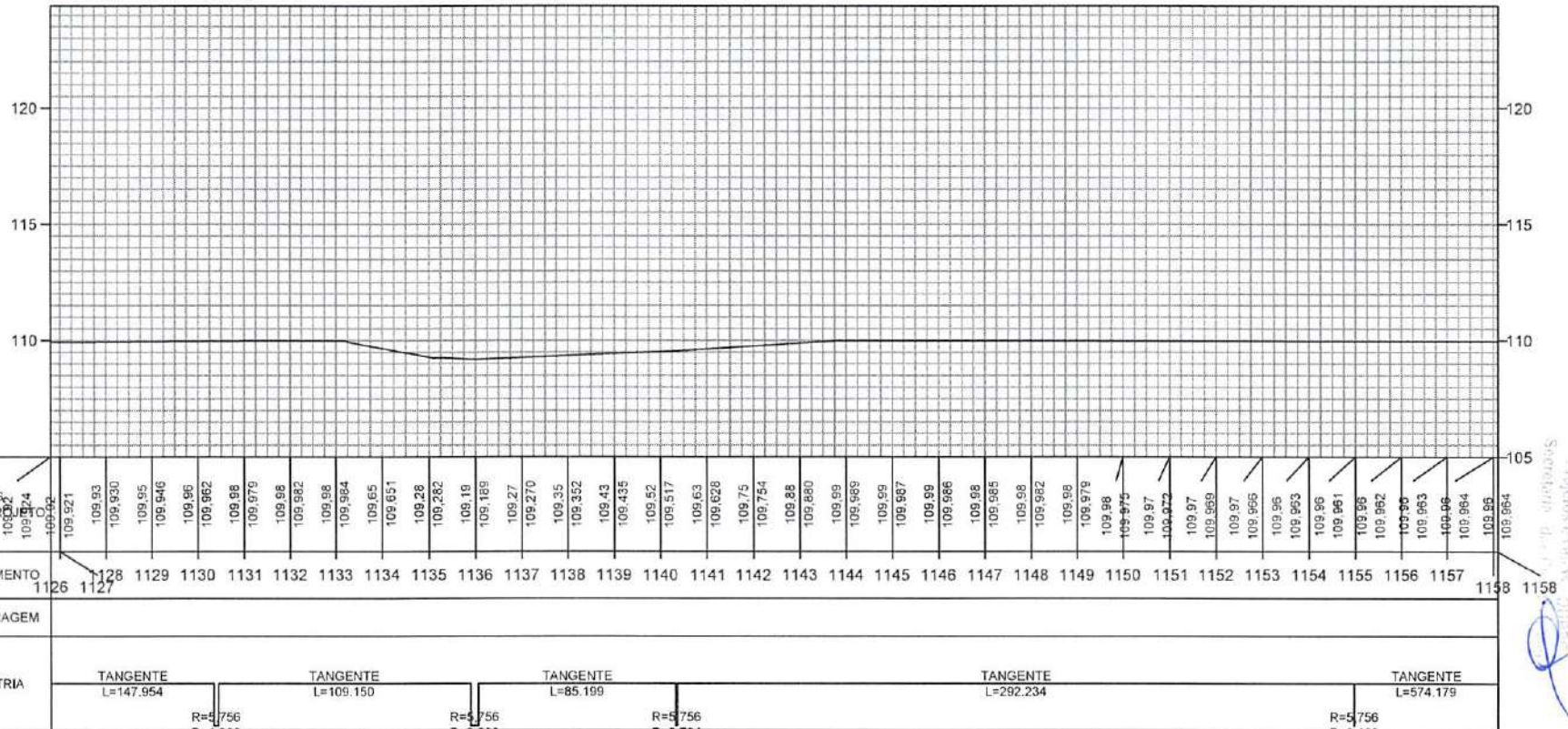
PERFIL ALINHAMENTO - 01
