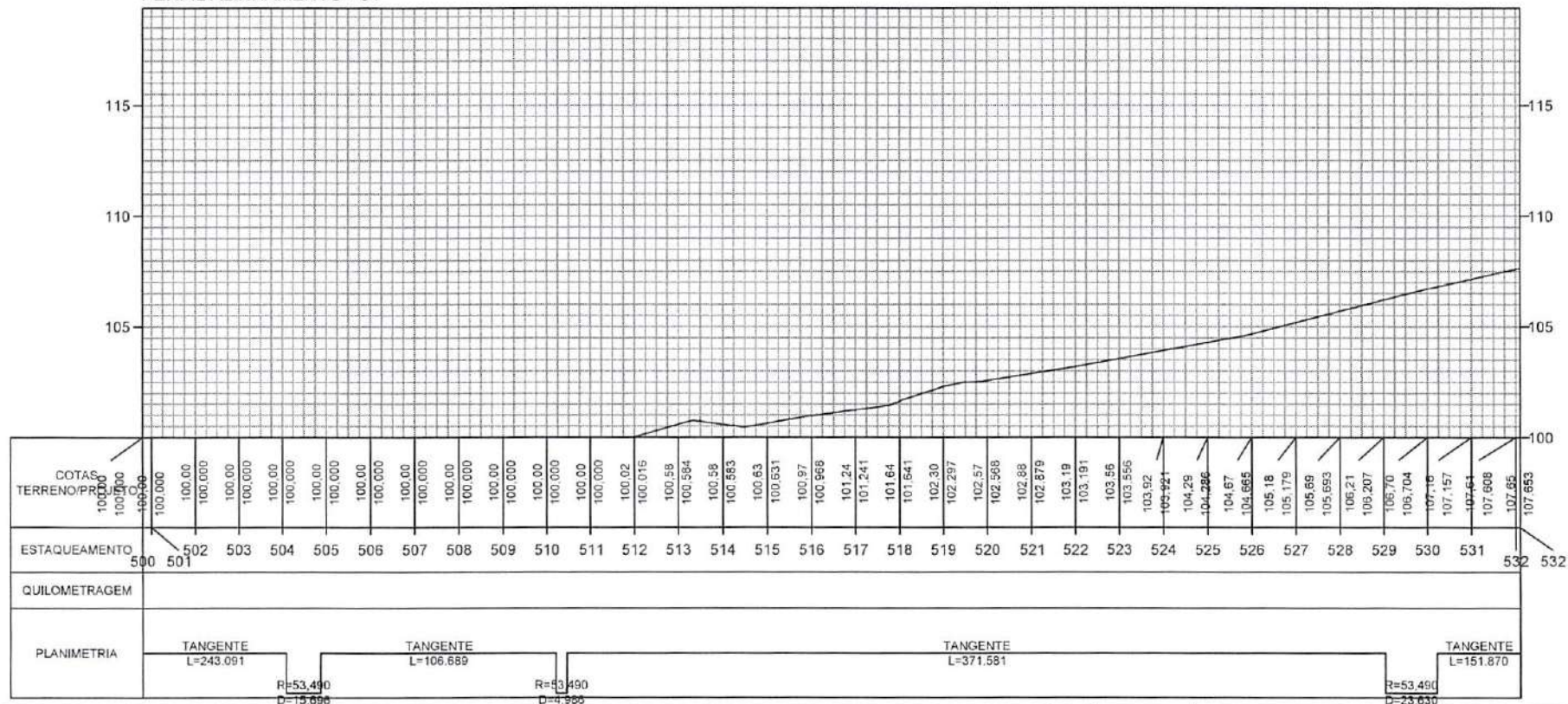
PERFIL ALINHAMENTO - 01
