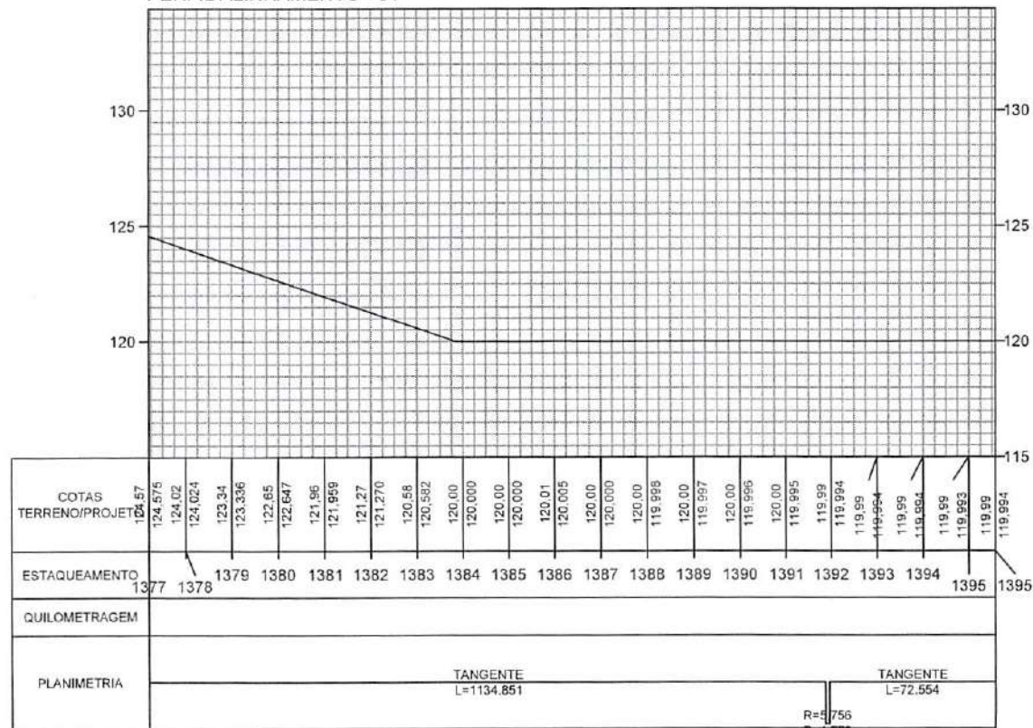
PERFIL ALINHAMENTO - 01
