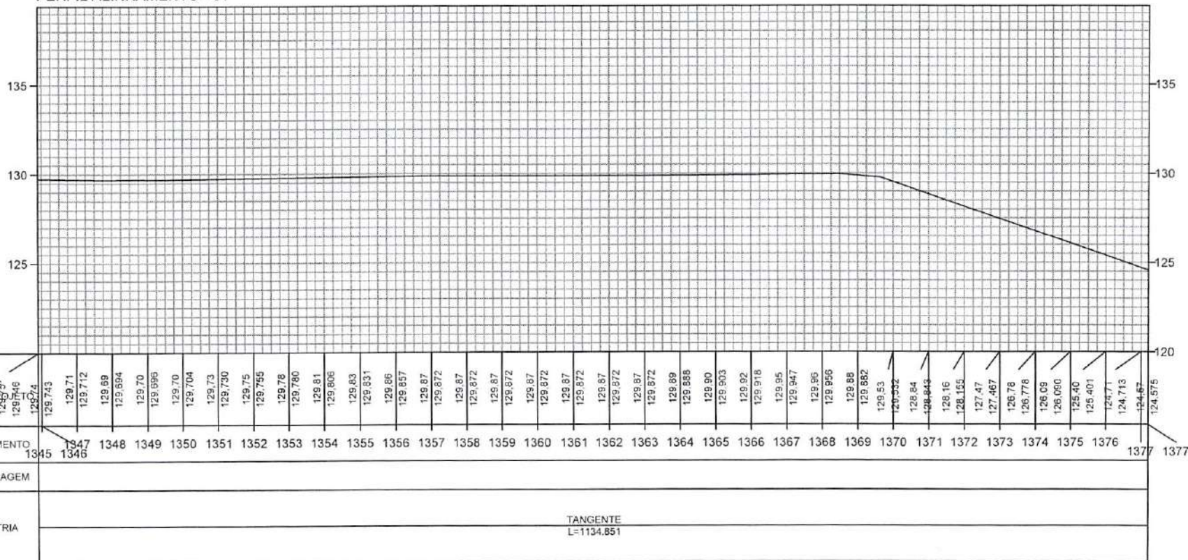
PERFIL ALINHAMENTO - 01
