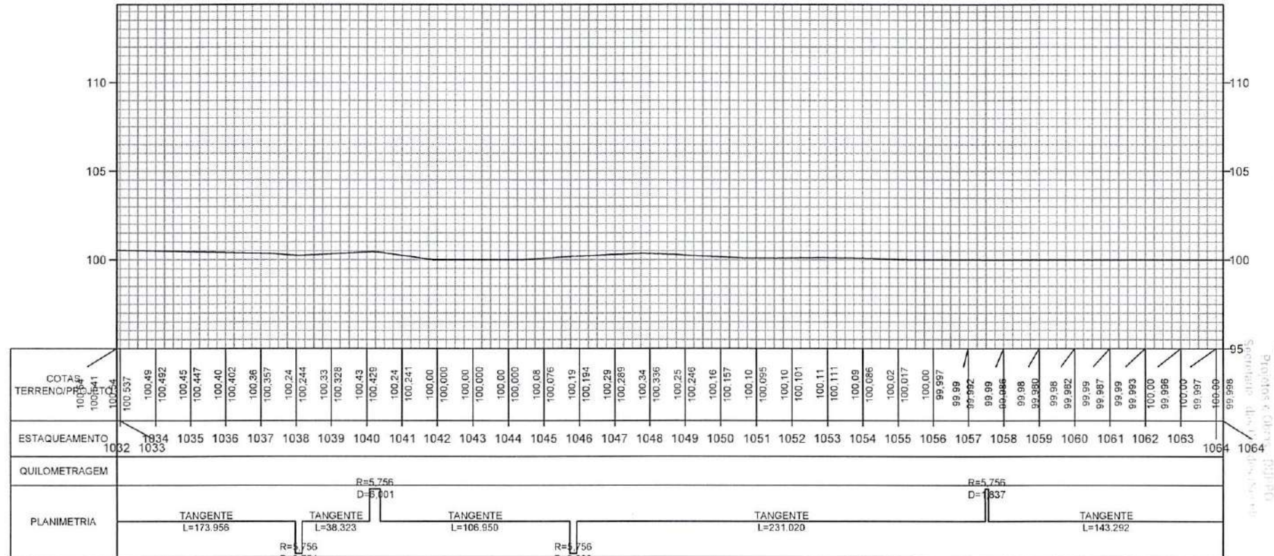
PERFIL ALINHAMENTO - 01
