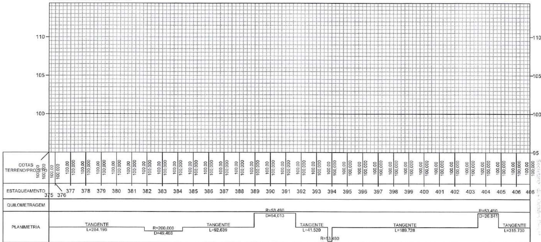
PERFIL ALINHAMENTO - 01
