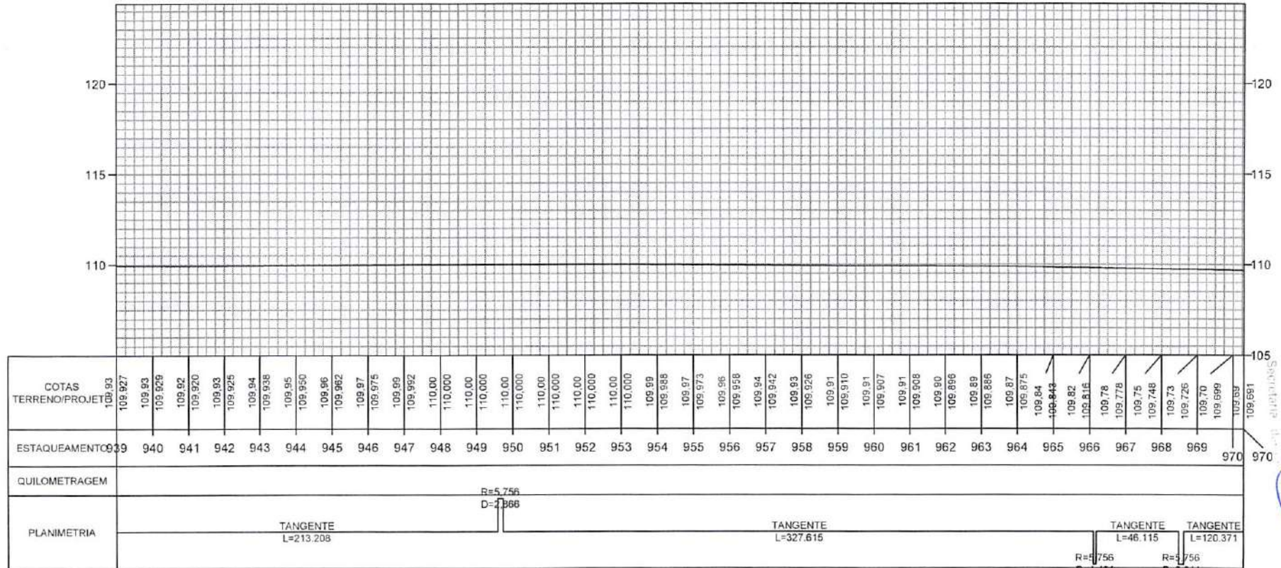
PERFIL ALINHAMENTO - 01
