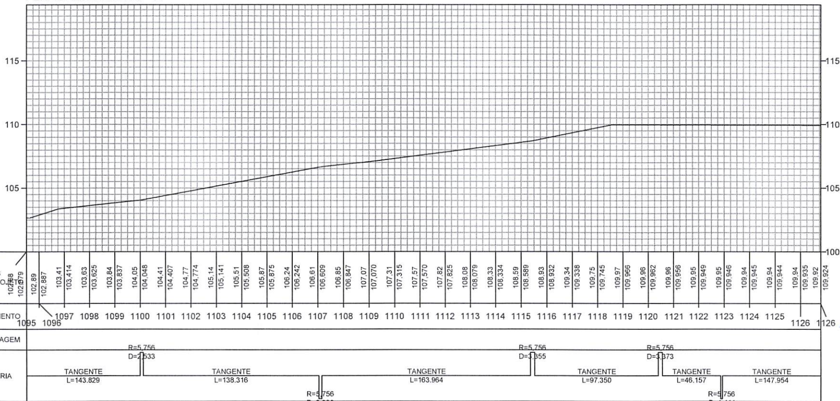
PERFIL ALINHAMENTO - 01
