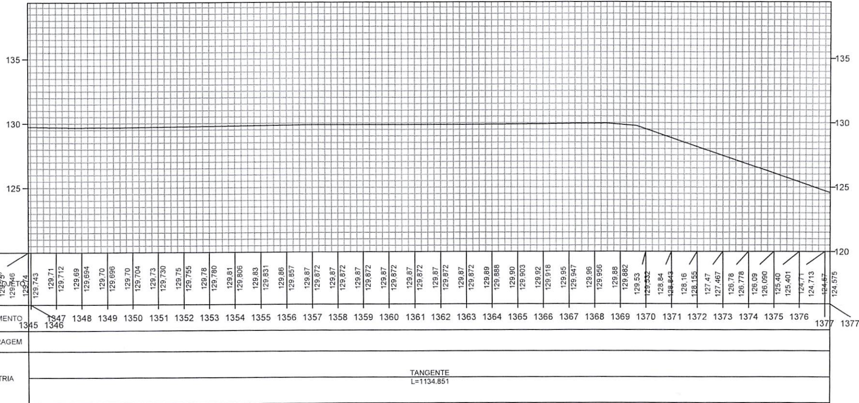
PERFIL ALINHAMENTO - 01
