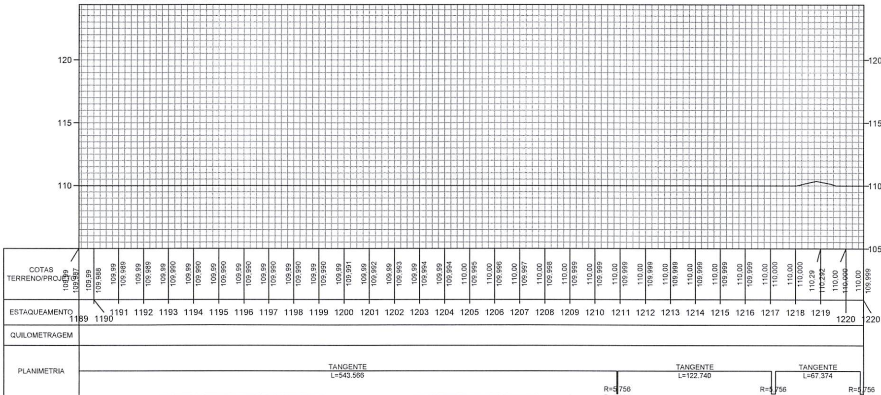
PERFIL ALINHAMENTO - 01
