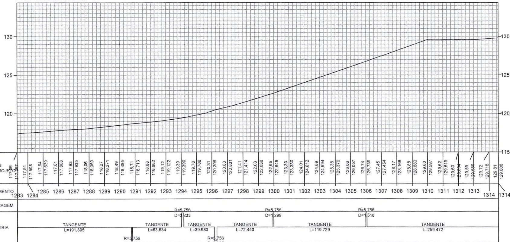
PERFIL ALINHAMENTO - 01
