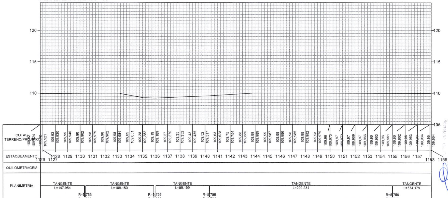
PERFIL ALINHAMENTO - 01
