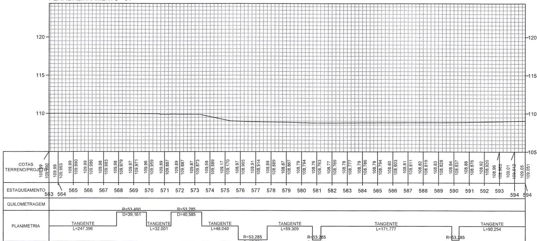
PERFIL ALINHAMENTO - 01
