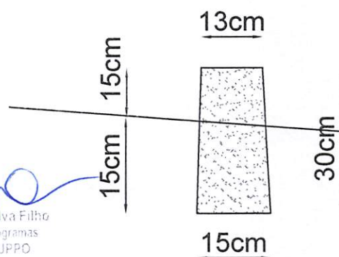
MEIO-FIO DE CONCRETO PRÉ-MOLDADO
