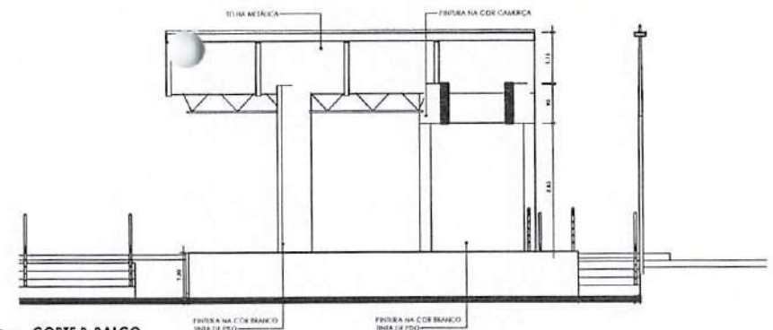
2 CORTE B-PALCO 1:75
