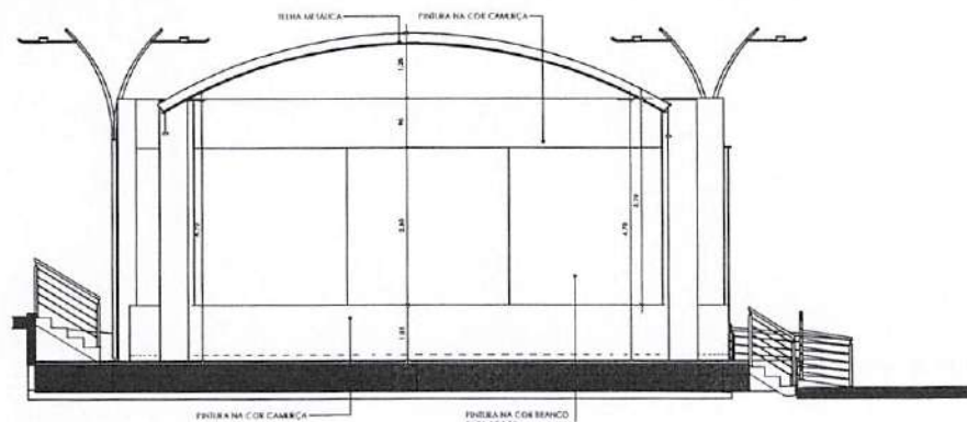
1 CORTE A-PALCO 1:75
