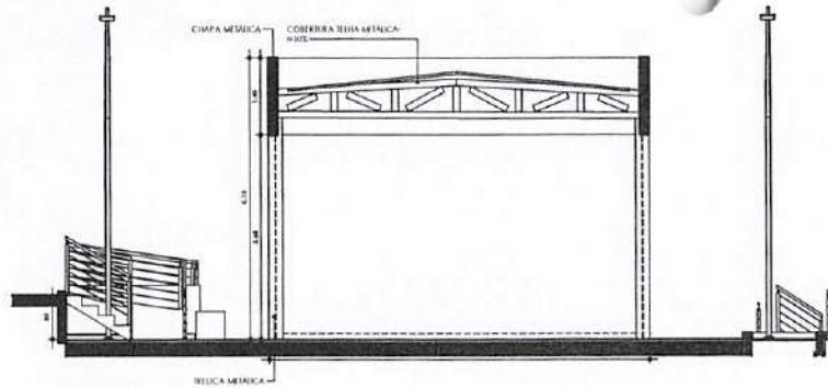
1 CORTE A-MERCADO 1:75
