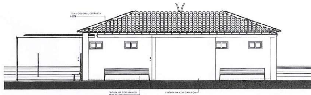
4 CORTE C-BANHEIROS
