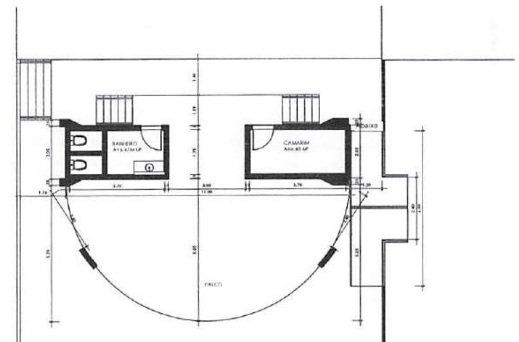
5 PLANTA BAIXA-PALCO EVENTOS 1:100
