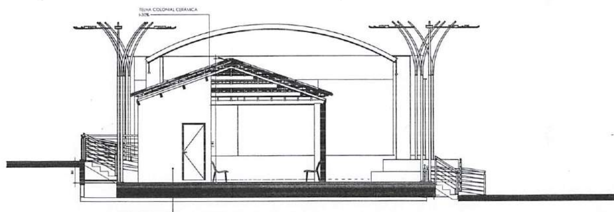
3 CORTE B-BANHEIROS 1 : 75
