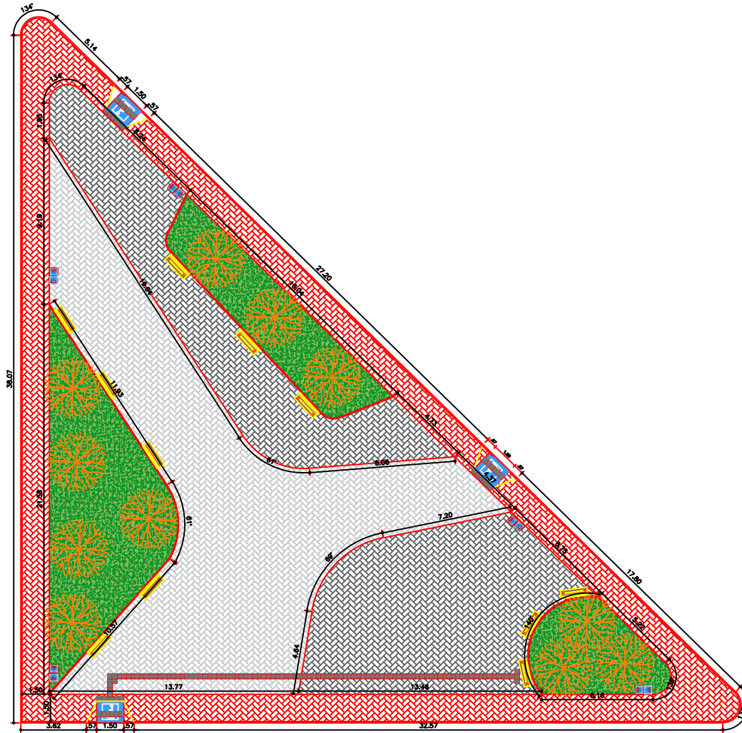
02 PLANTA BAIXA DE CONSTRUÇÃO Escala: 1/25
