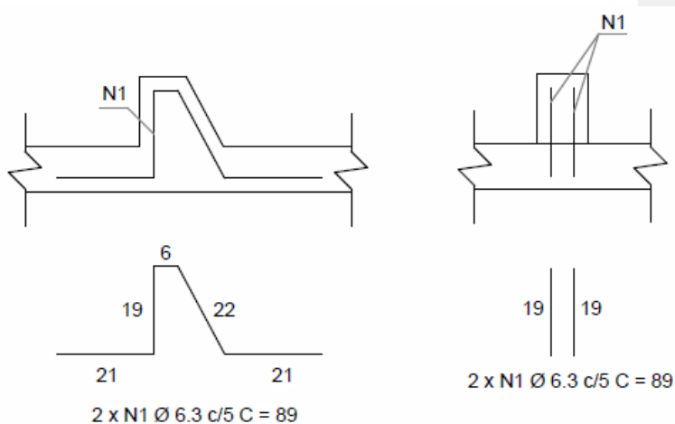
Corte C-C'
