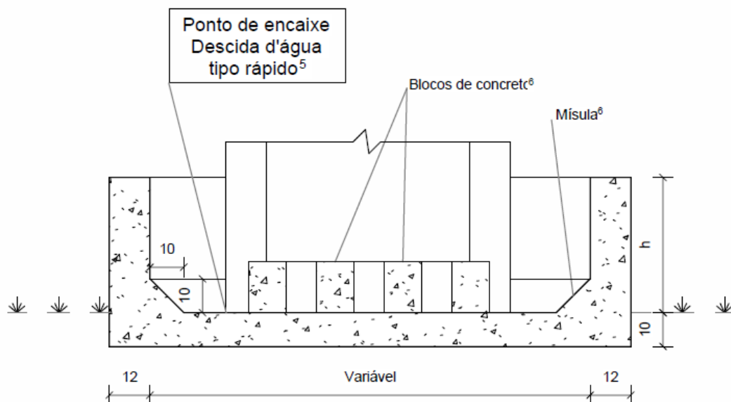
Corte B-B'
