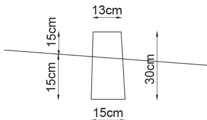
MEIO-FIO DE CONCRETO PRÉ-MOLDADO
