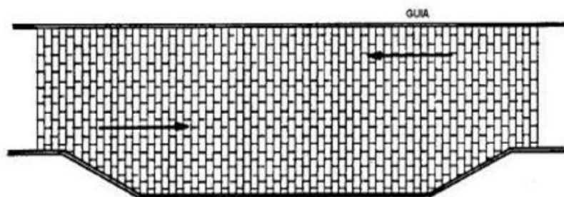
Figura 08. Trecho Reto, com Alargamento para Estacionamento
